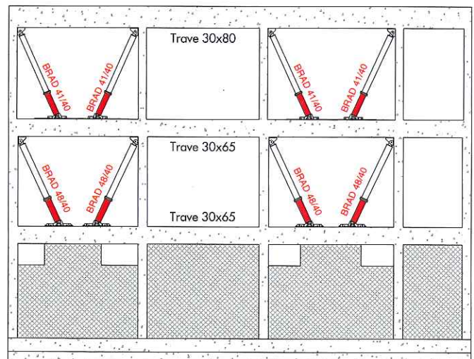
TELAIO 1X
